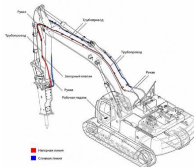
Рис. 1. Экскаватор Hitachi ZX-180 LC-3
